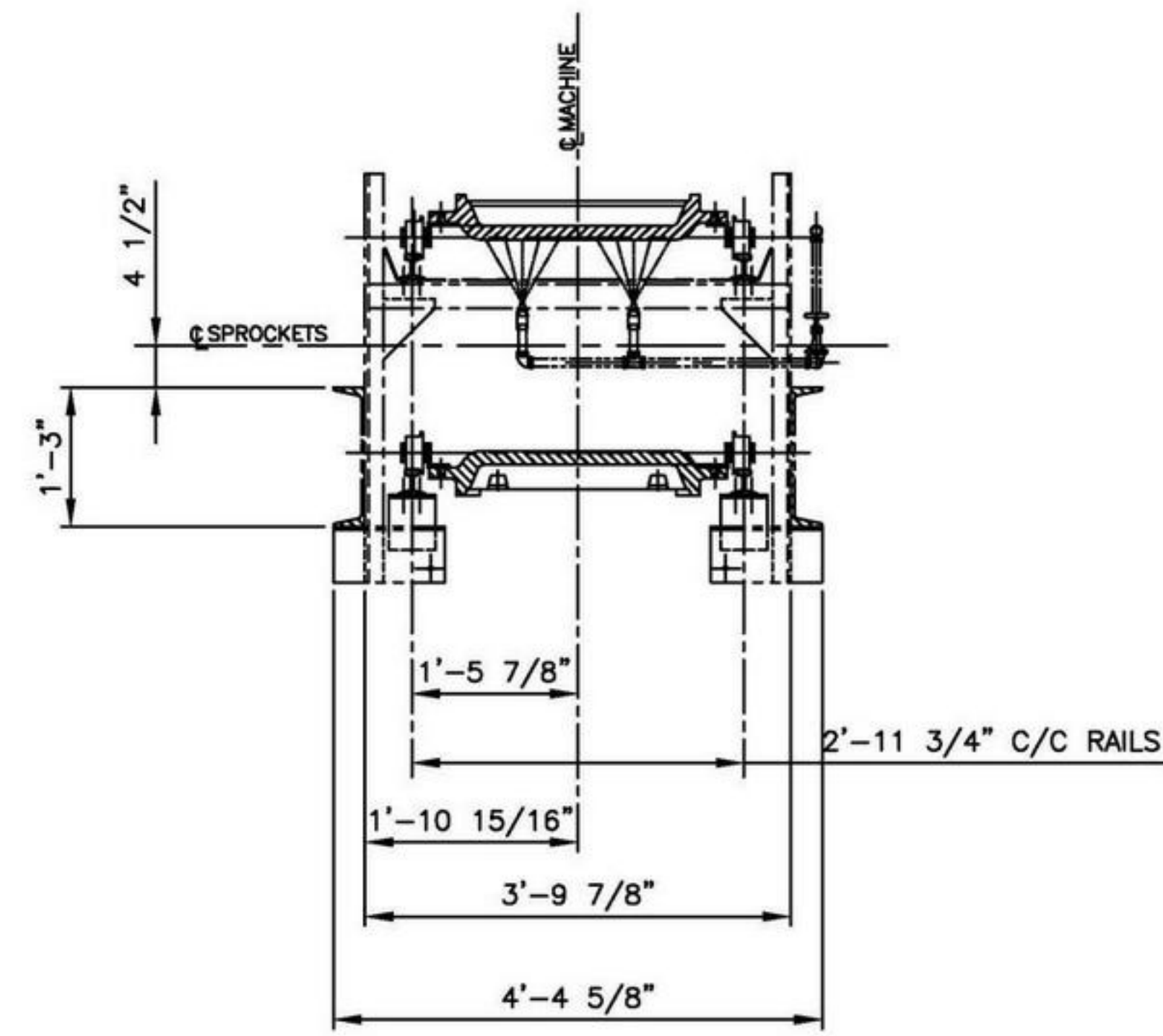
ENL. SECTION A-A
