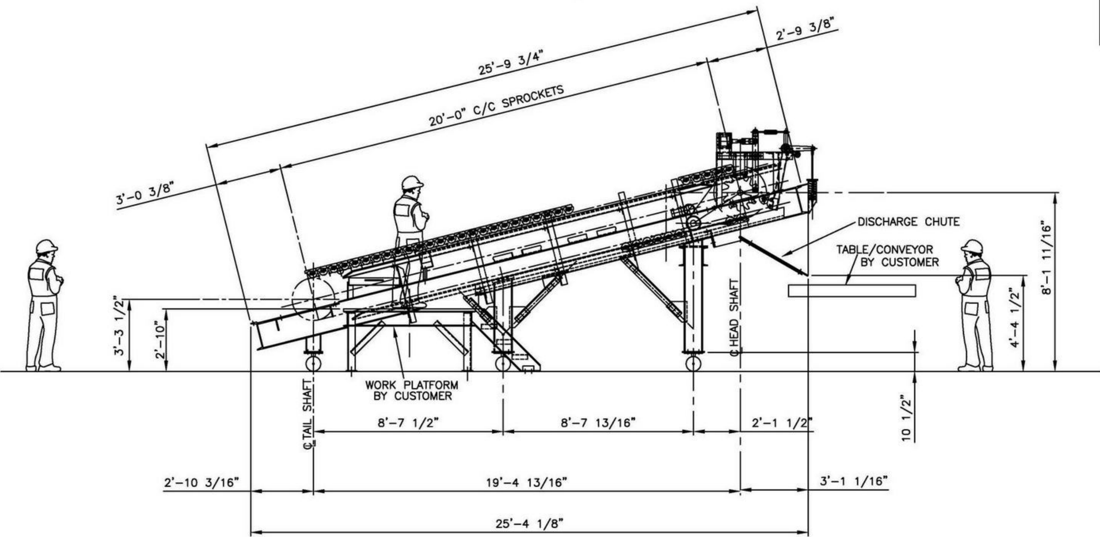
ENL. SECTION A-A
